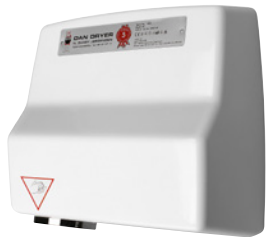
DAN DRYER AE Berührungsfrei – mit IR Sensor Aluminiumgehäuse Trocknungszeit: 20-25 Sek. 5 Jahre Garantie, inkl. Vandalismus 230 V, 50/60 Hz, 2360 W H: 313 mm, B: 311 mm, T: 178 mm Art.-Nr. 261 – weiß pulverlackiert
