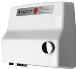
DAN DRYER AA Modell mit Druckknopf Aluminiumgehäuse Trocknungszeit: 20-25 Sek. 5 Jahre Garantie, inkl. Vandalismus 230 V, 50/60 Hz, 2360 W H: 313 mm, B: 311 mm, T: 201 mm Art.-Nr. 100 – weiß pulverlackiert
