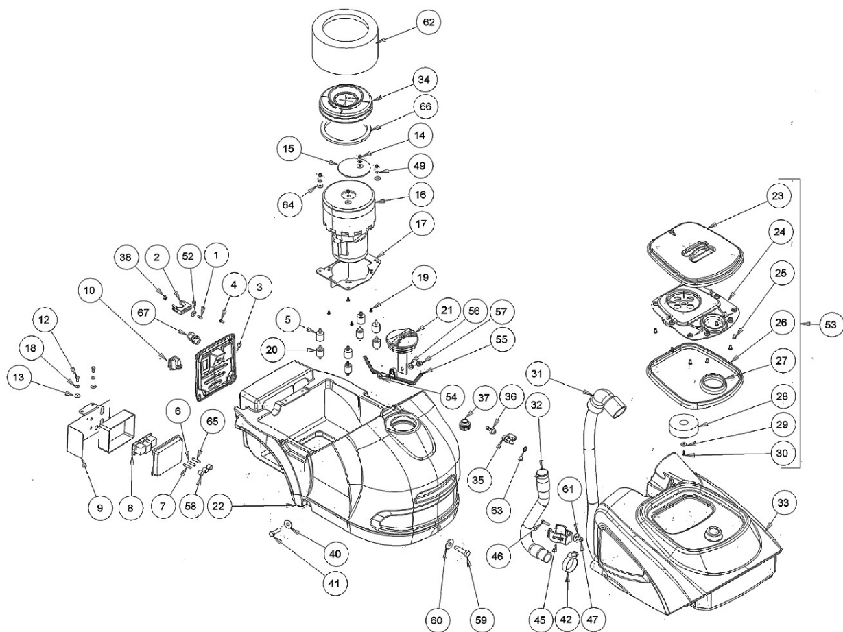
Abb. / Fig. 5: Ersatzteilzeichnung 1/ Spare parts drawing 1
