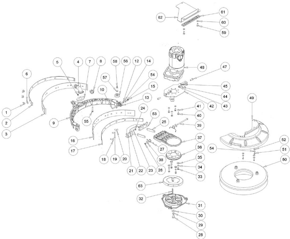
Abb. / Fig. 7: Ersatzteilzeichnung 3 / Spare parts drawing 3
