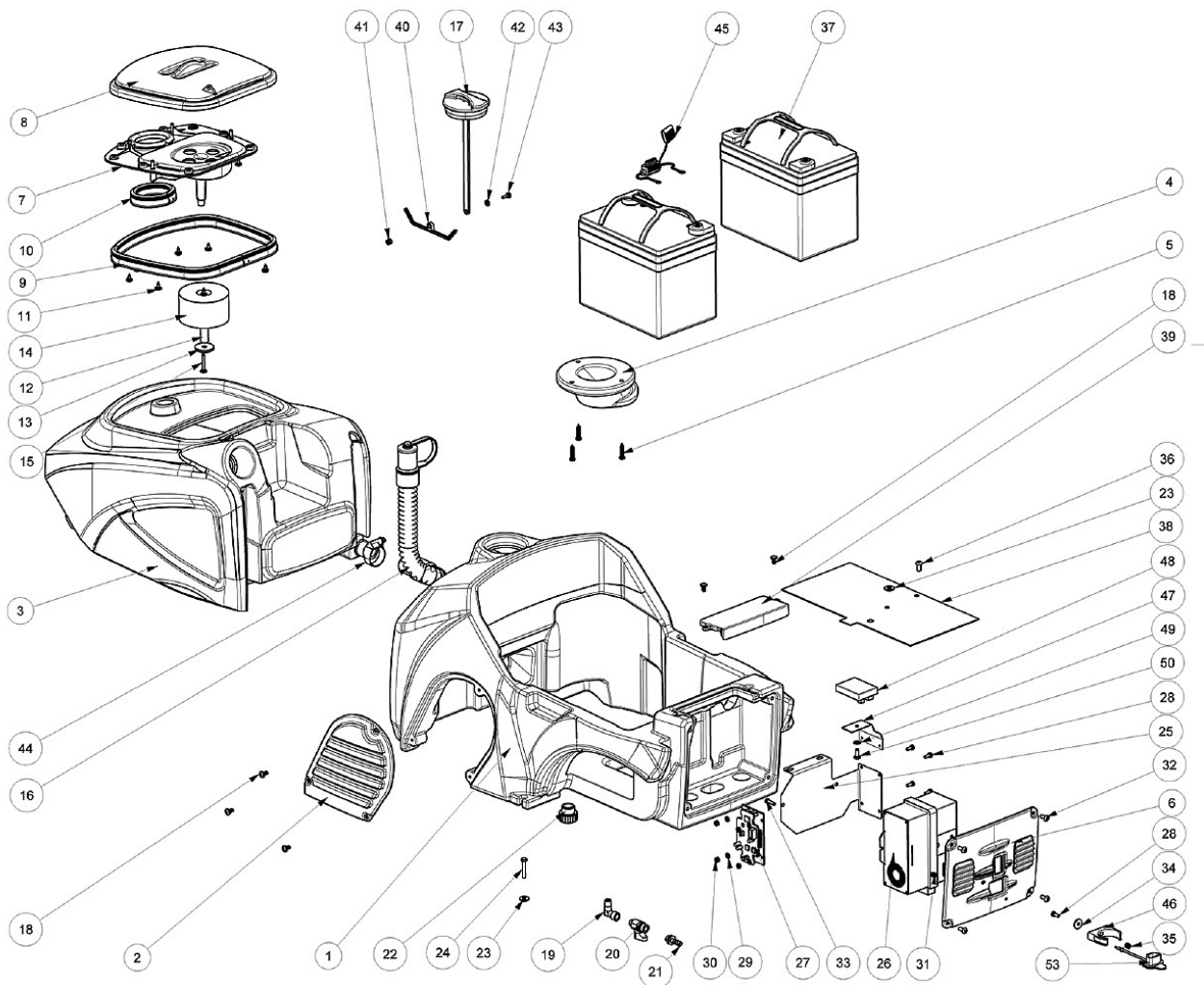
Abb. / Fig. 11: Ersatzteilzeichnung 3 / Spare parts drawing 3
