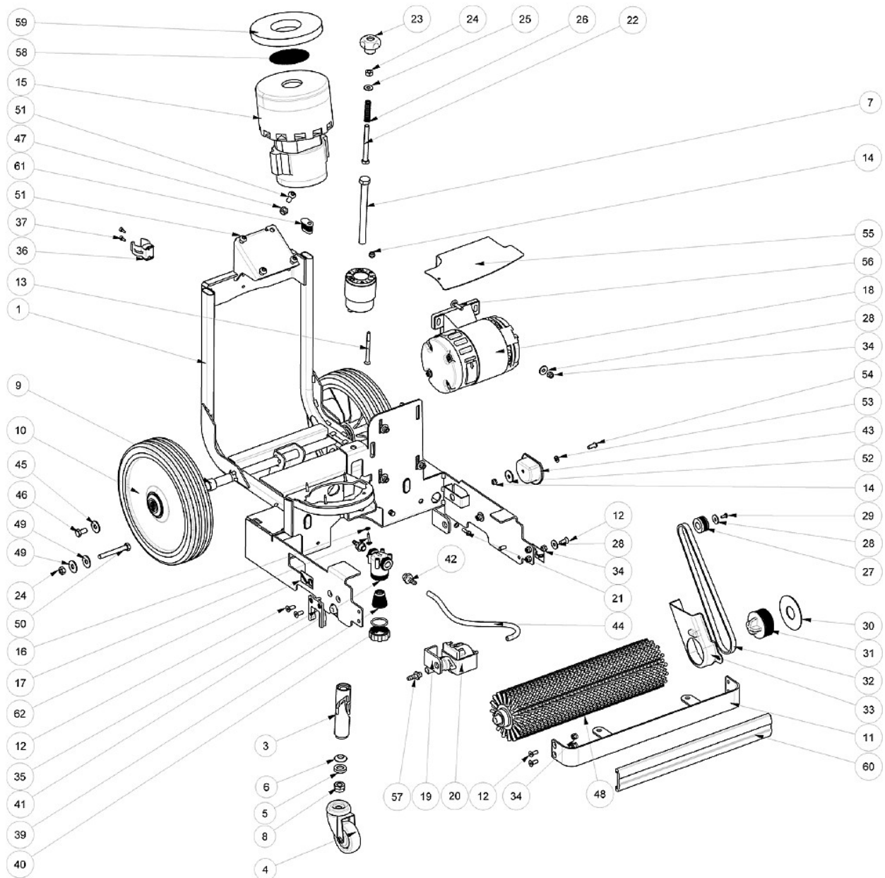
Abb. / Fig.. 10: Ersatzteilzeichnung 2 / Spare parts drawing 2
