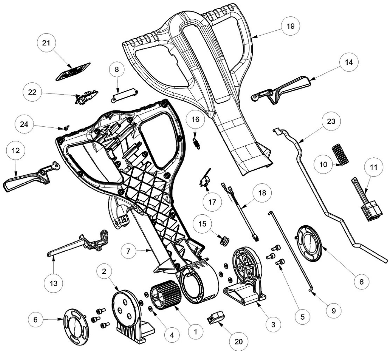
Abb. / Fig. 12: Ersatzteilzeichnung 4 / Spare parts drawing 4
