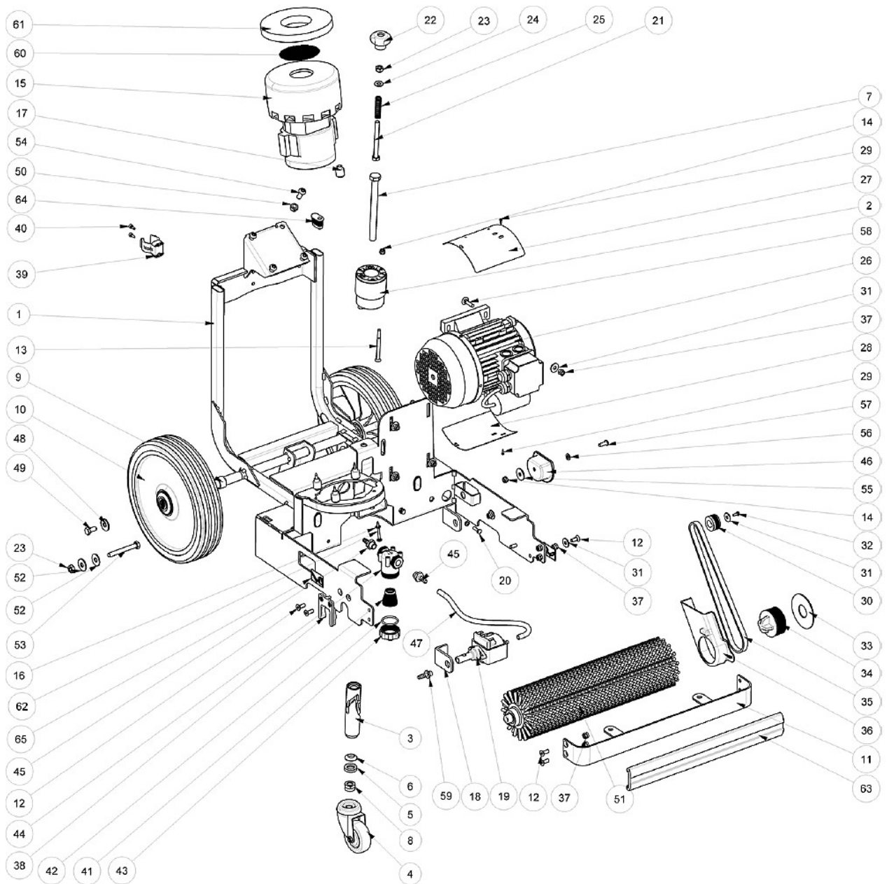
Abb. / Fig. 14: Ersatzteilzeichnung 2 / Spare parts drawing 2
