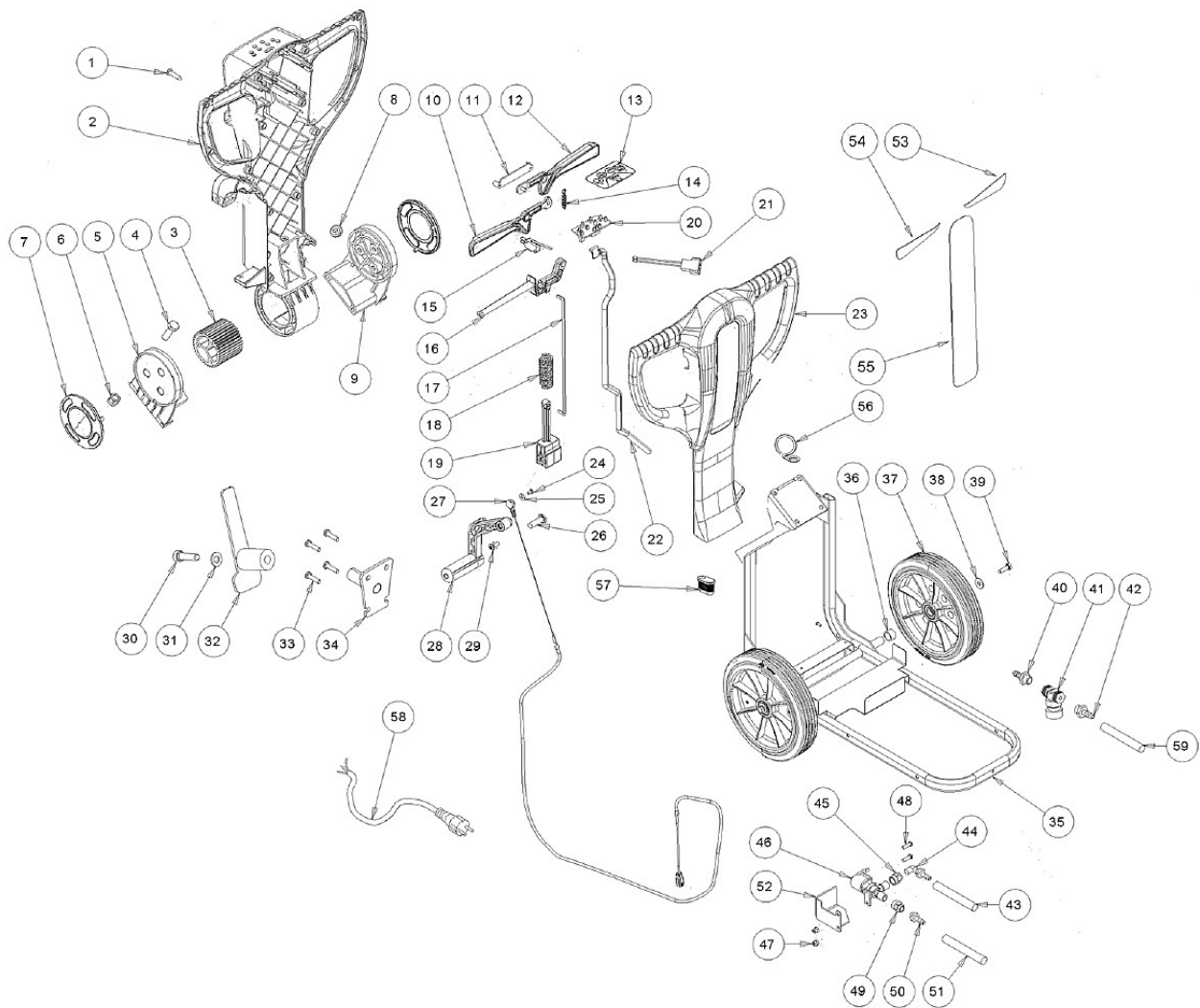
Abb. / Fig. 8: Ersatzteilzeichnung 4 / Spare parts drawing 4
