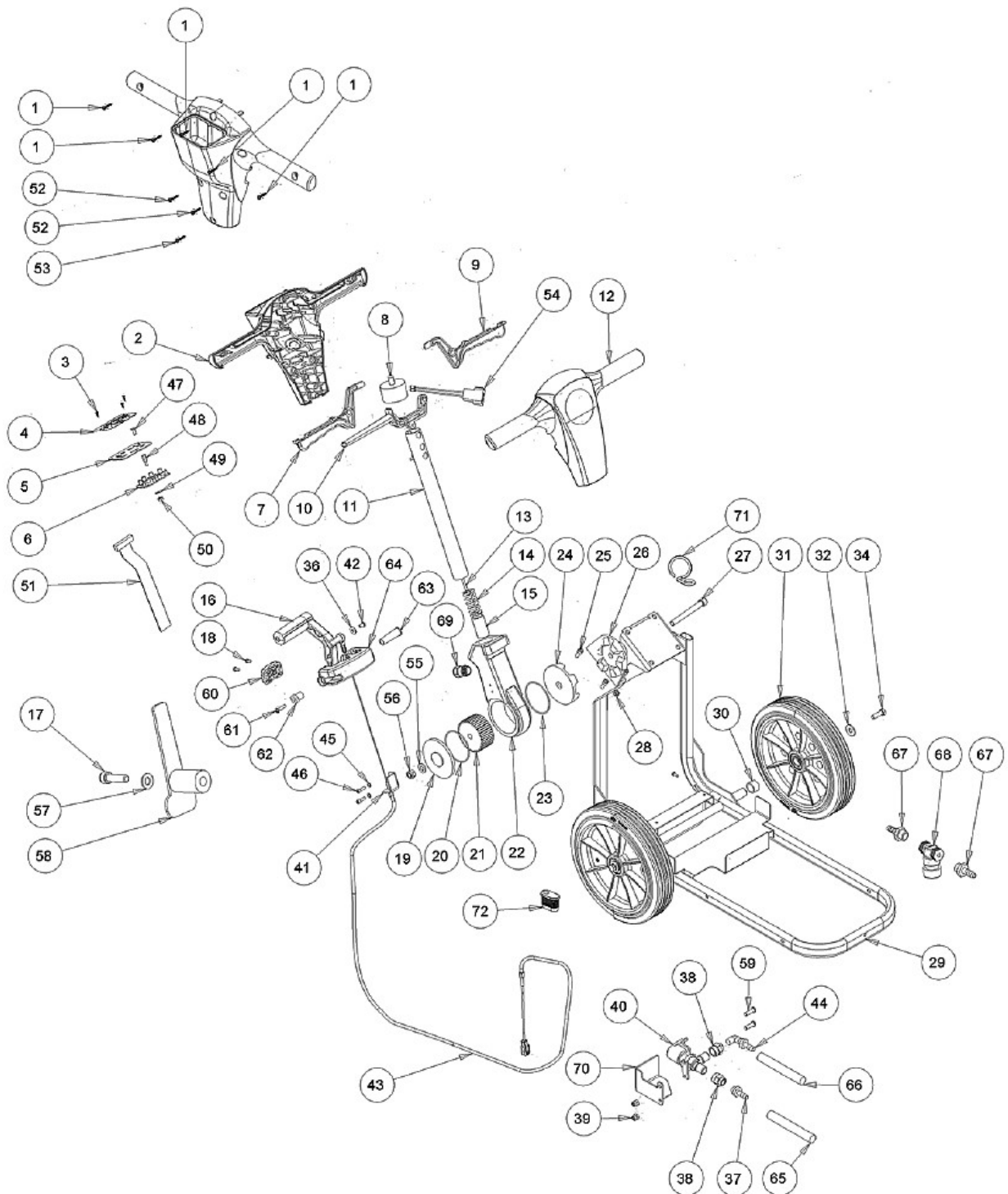
Abb. / Fig. 6: Ersatzteilzeichnung 2 / Spare parts drawing 2
