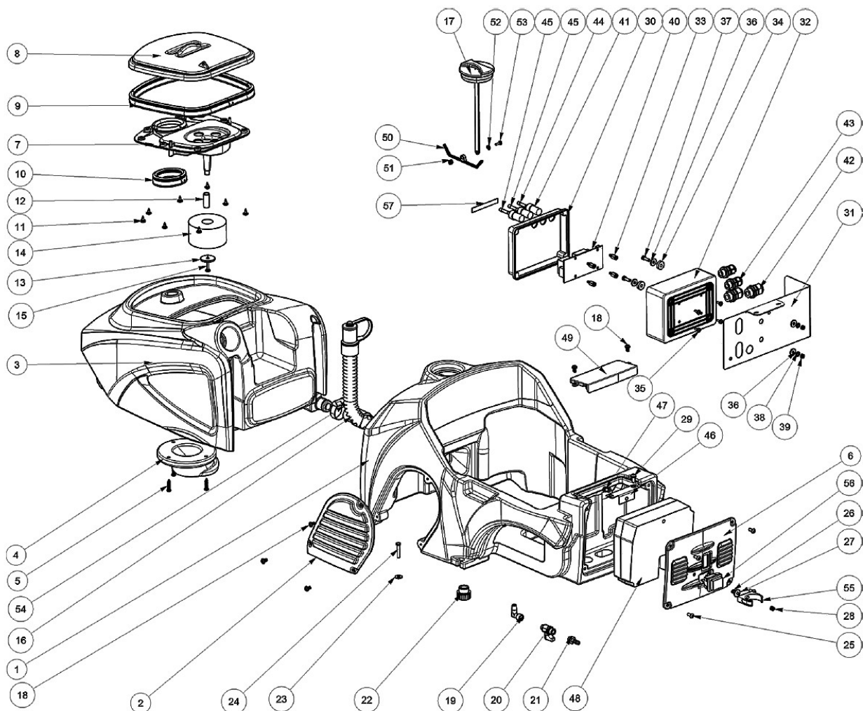
Abb. / Fig. 15: Ersatzteilzeichnung 3 / Spare parts drawing 3
