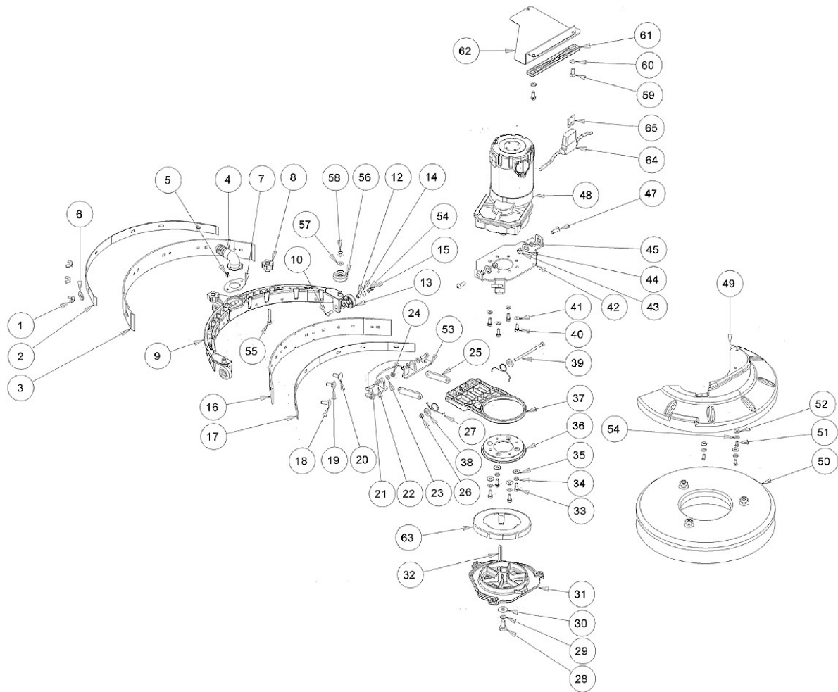
Abb. / Fig. 3: Ersatzteilzeichnung 3 / Spare parts drawing 3
