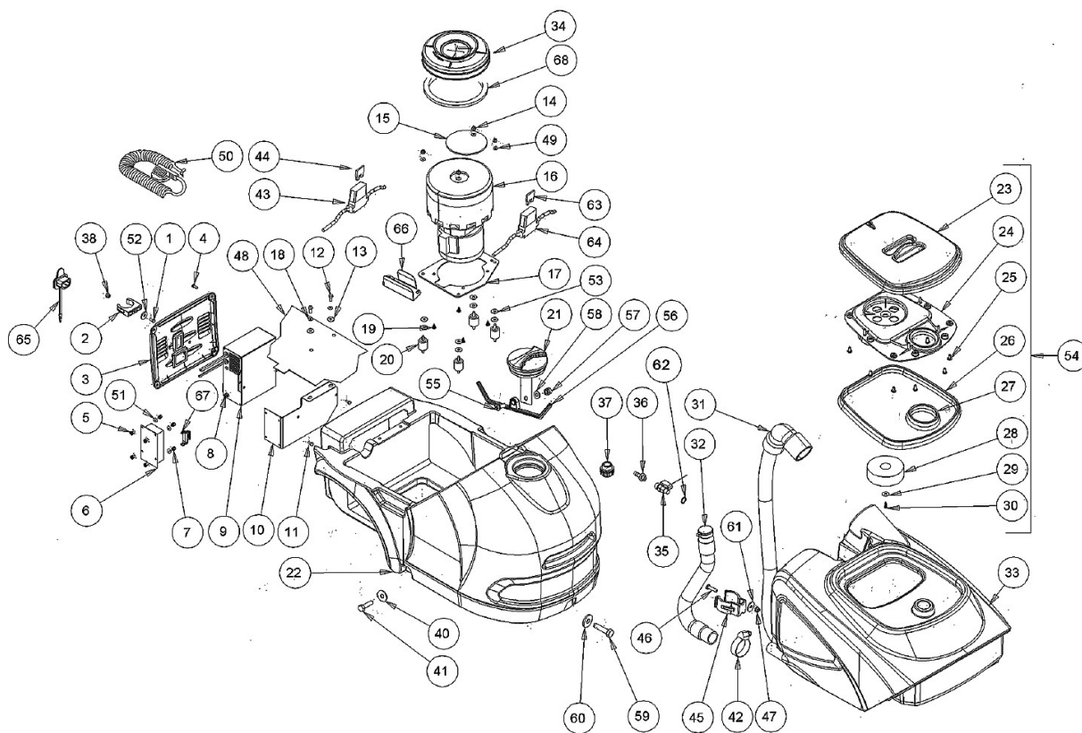
Abb. / Fig. 1: Ersatzteilzeichnung 1 / Spare parts drawing 1
