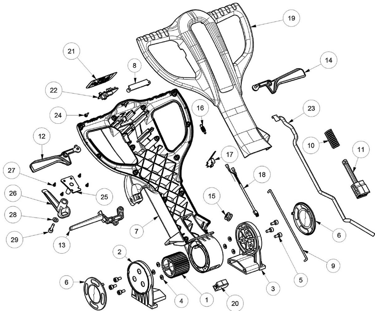
Abb. / Fig. 16: Ersatzteilzeichnung 4 / Spare parts drawing 4
