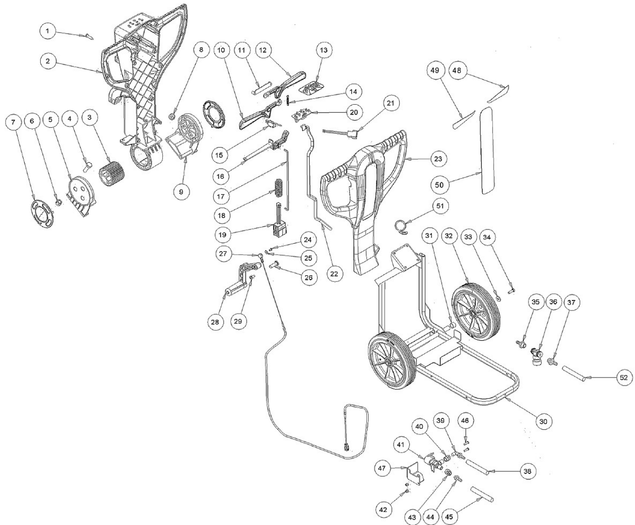
Abb. / Fig. 4: Ersatzteilzeichnung 4 / Spare parts drawing 4
