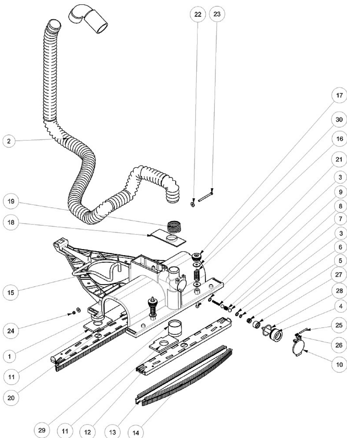
Abb. / Fig. 13: Ersatzteilzeichnung 1 / Spare parts drawing 1
