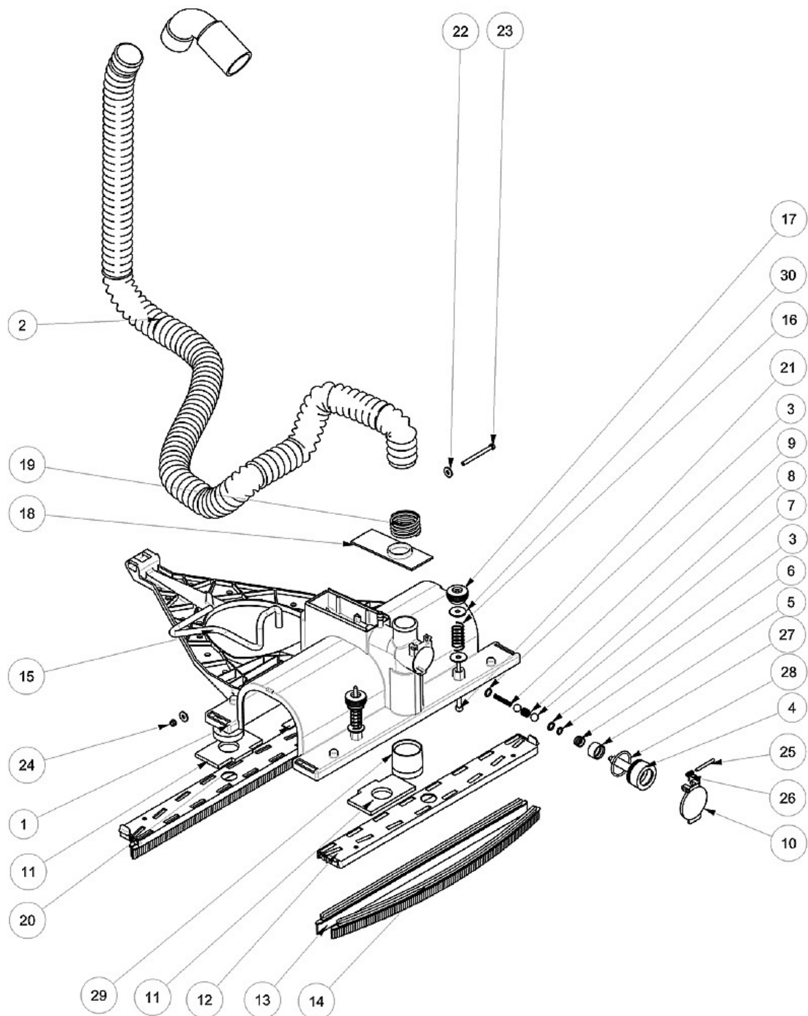
Abb. / Fig. 9: Ersatzteilzeichnung 1 / Spare parts drawing 1
