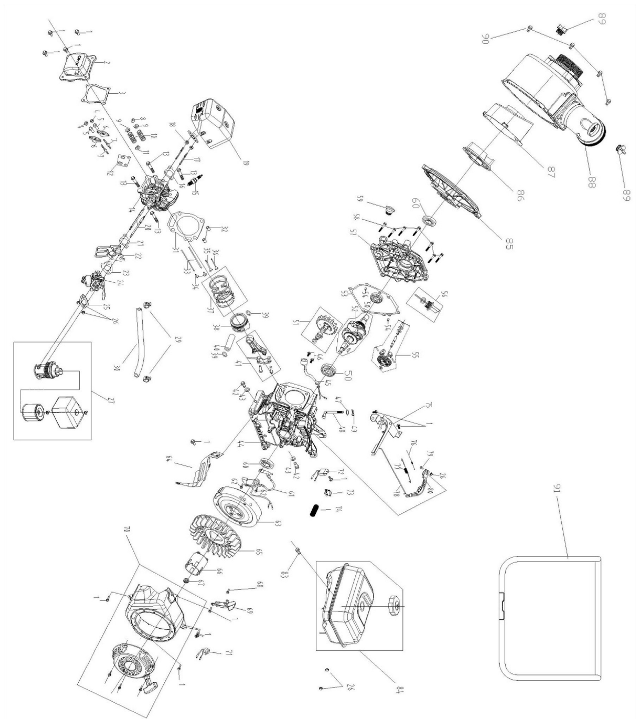
Abb. / Fig. 1: Ersatzteilzeichnung SWP 80 / Spare parts drawing SWP 80
