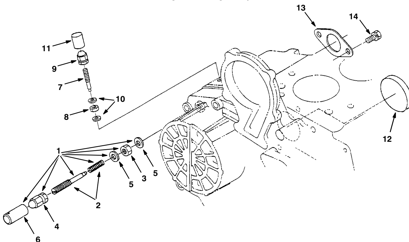
Fig. 18 – Idling Group
