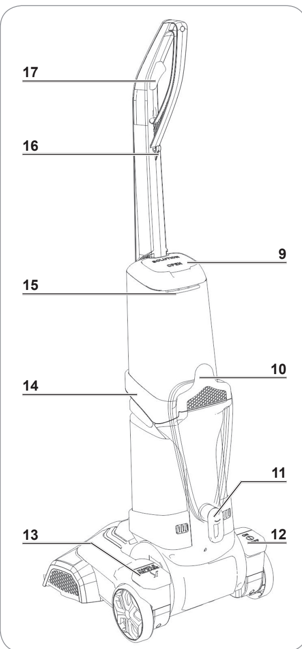
Face arrière
