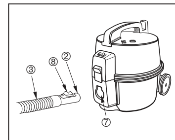
Abb. 3 Anbringen des Schlauches
