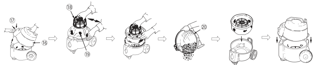
Abb. 12 Staubentfernung
