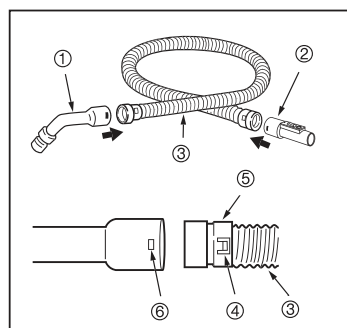
Abb. 2 Schlauchmontage
