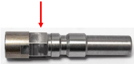
Verdrehsicherung am Stecknippel
