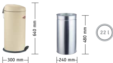
Kunststoff-Fußtritt Plastic pedal
